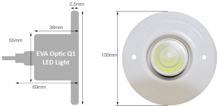
Zij-aanzicht Q1.
